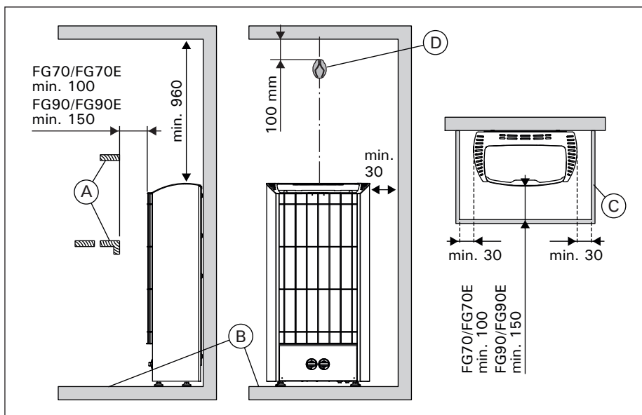
Figure 6. Safety distances (all dimensions in millimeters) Abbildung 6. Sicherheitsmindestabstände (alle Abmessungen in Millimetern)
