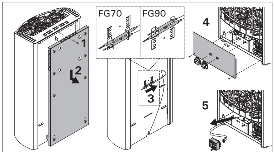
Figure 11. Replacing the thermostat Abbildung 11. Austauschen des Thermostats
