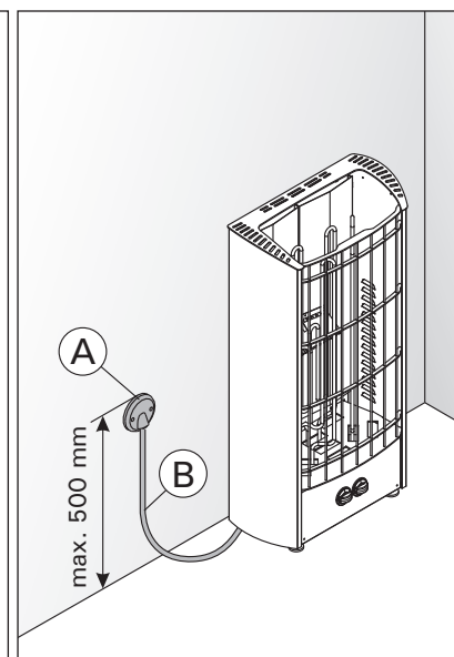
Figure 7. Cables Abbildung 7. Kabel
