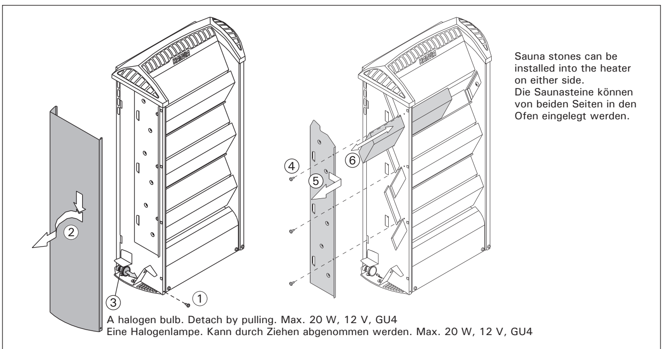
Figure 1. Changing a bulb of the heater light and installation of sauna stones Abbildung 1. Auswechseln der Glühbirne der Ofenlampe und Aufschichten der Saunasteine
