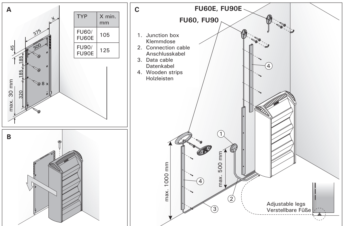
Figure 7. Location of the heater mounting rack and connecting the heater Abbildung 7. Platz des Montagegestells des Saunaofens und Anschluss des Ofens
