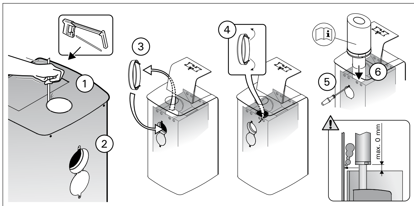
Figure 11. Connecting the stove to a Harvia steel chimney (all dimensions in millimeters) Abbildung 11. Anschluss des Ofens an einen Harvia-Edelstahlschornstein (alle Abmessungen in Millimetern)
