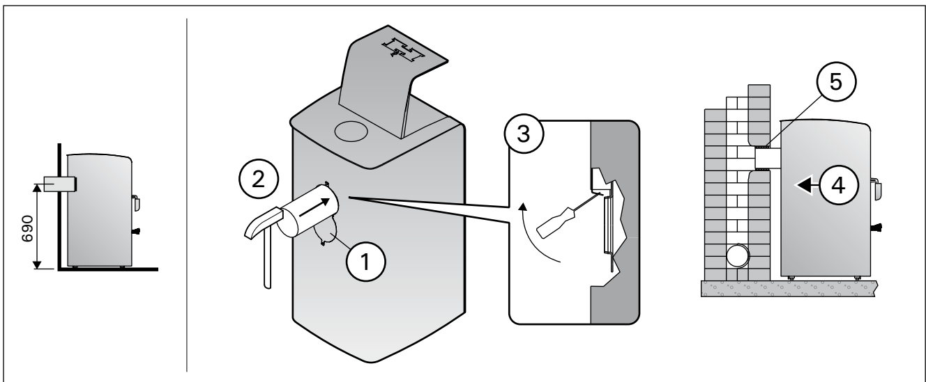
Figure 9. Connecting the stove to a masonry flue via the rear connection opening (all dimensions in millimeters) Abbildung 9. Anschluss des Ofens an einen gemauerten Rauchfang über die hintere Anschlussöffnung (alle Abmessungen in Millimetern)
