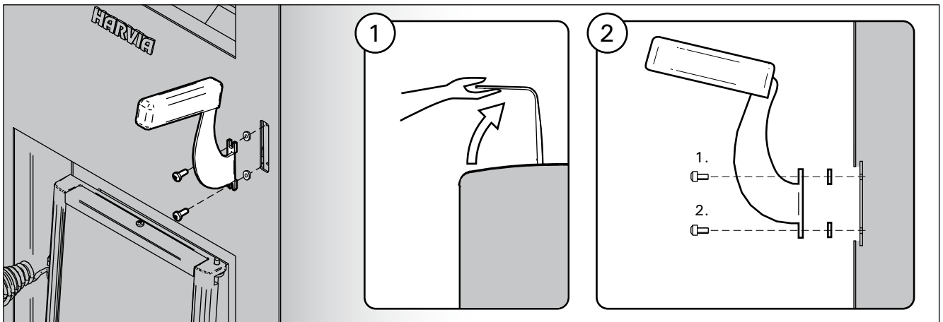
Figure 12. Installing the handle Abbildung 12. Montage der Griff
