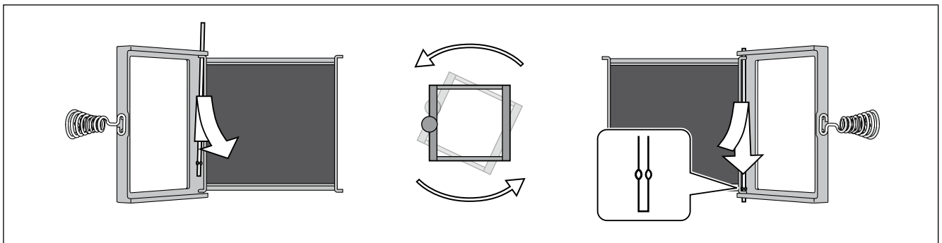
Figure 13. Changing the opening direction of the stove door Abbildung 13. Änderung der Öffnungsrichtung der Ofentür
